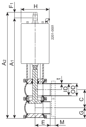
Abbildung 1. Absperrventil
